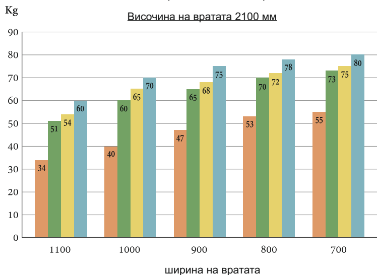
Схема товароносимост, кг за врата
