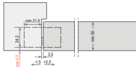
Схема товароносимост 3 панти
