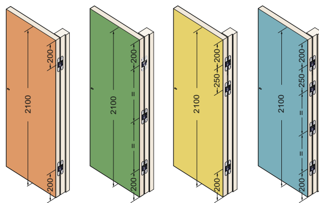
Схема товароносимост, кг за врата Височина на вратата 2100 мм
